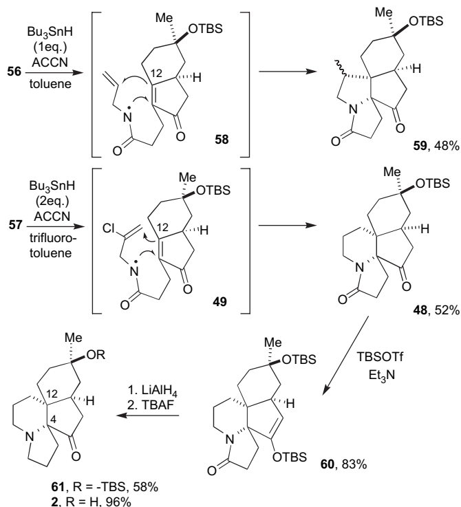
Scheme 14.
